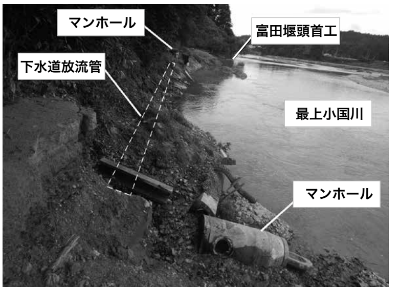
浸食、流出した下水道の放流管
