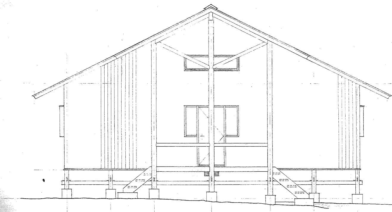
A 立面图
