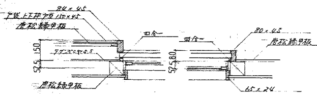
詳細図 1:20
