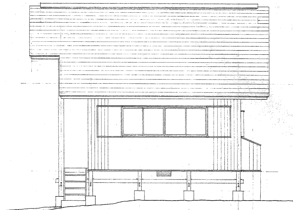
B 立 面 図
