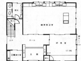
1階平面図
