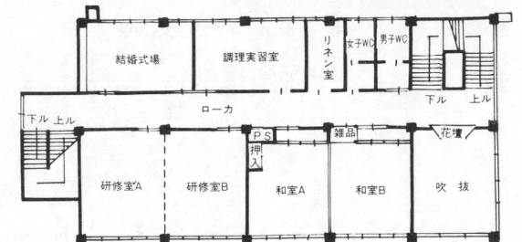
▲ (二階平面図)
