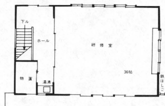
2階平面図
