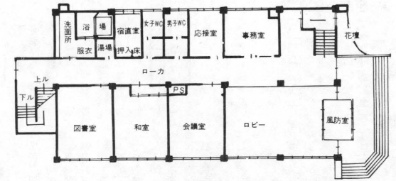
▲ (一階平面図)
