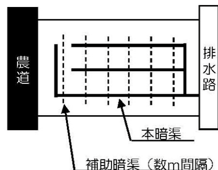
【暗渠排水のイメージ】
